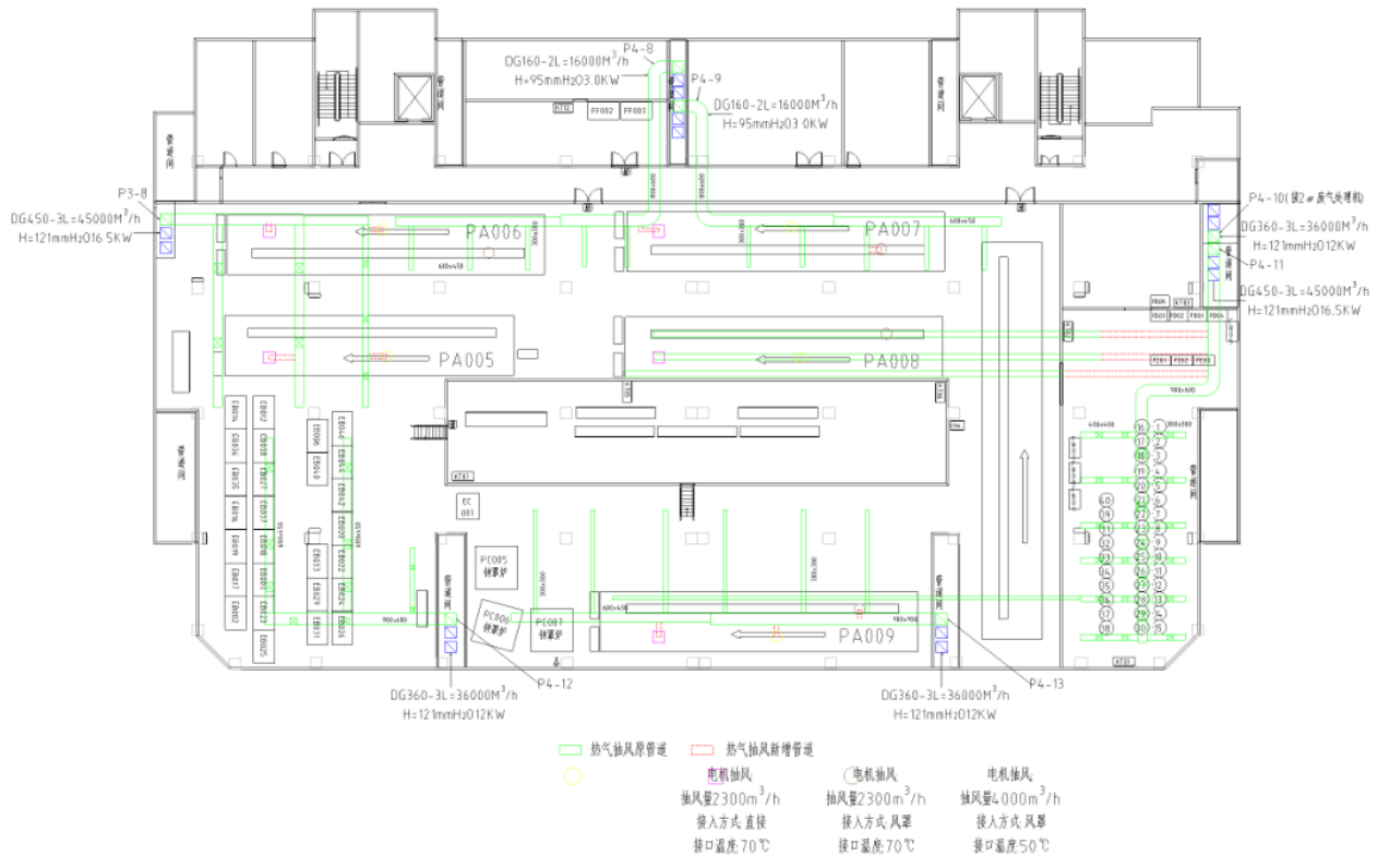
烧炉车间3#楼四楼热气抽风修改后平面图
