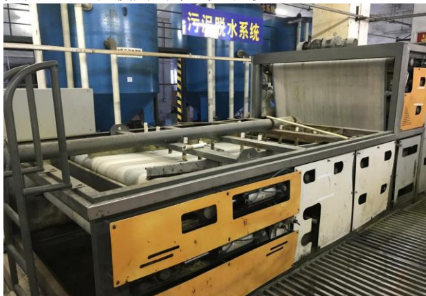
附图 3:正在使用的带式压泥机
