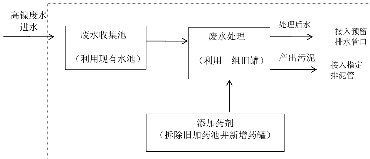
风华高科高镍废水预处理项目工艺流程图
